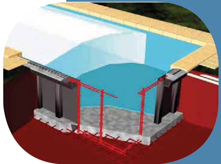
Coupe et présentation des bétons et ferrillages parois et fond
